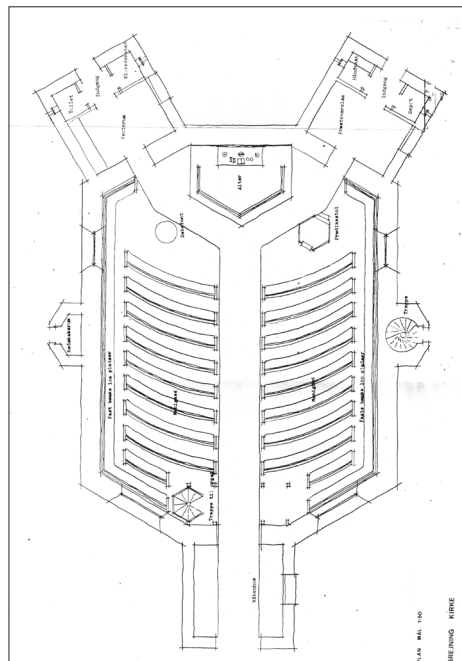
Brejning Kirke . Tegning af grundplan 1941.
